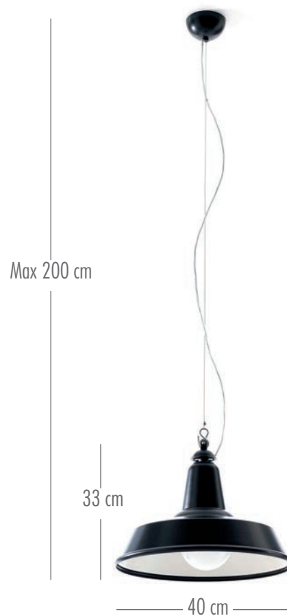
GIRONA S40 1xE27 Max 70W
